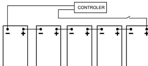
Figura 1-10 Diagrama schematică a cablajului acumulatorului
