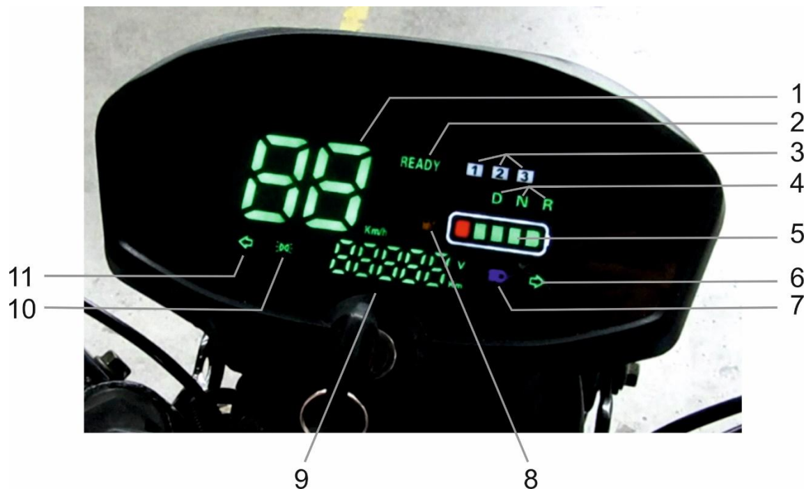
Figura 1-1 Afişaj bord
