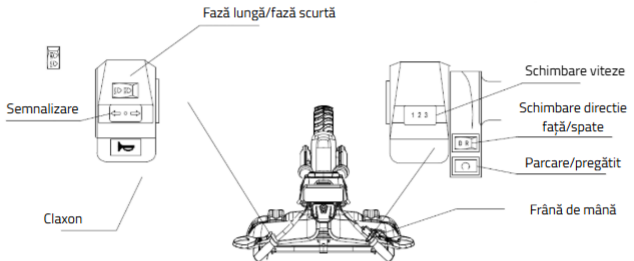
Mâner stânga
